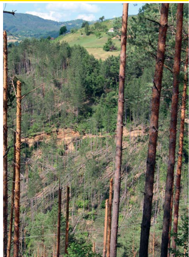
Над 60 % е падналата дървесина в м. Пункови колиби, ГСУ - Неделино
